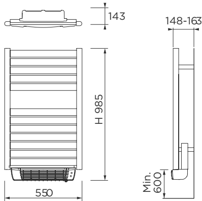
Die Maße sind in mm angegeben
