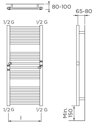
Die Maße sind in mm angegeben
