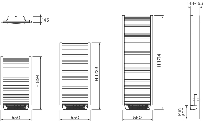
Die Maße sind in mm angegeben
