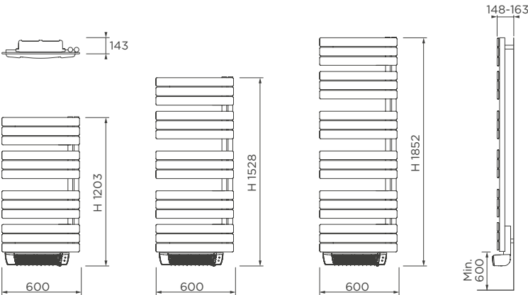
Die Maße sind in mm angegeben
