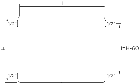
Vorderansicht
