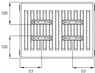
Draufsicht
