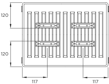
Draufsicht
