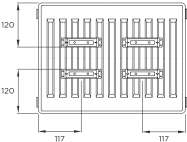
Draufsicht
