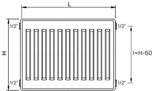
Rückansicht mod. 20-30
