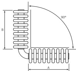
Seitenanschluss
